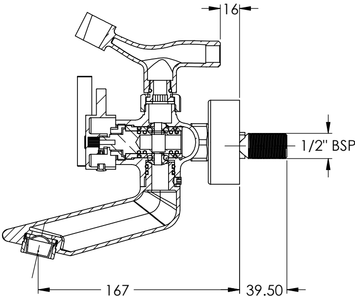
SECTION D-D SCALE 1 : 3.1
